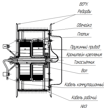
Рис.2 Устройство кабельного барабана
