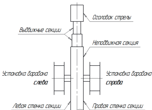
Рис.4 Стороны установки
