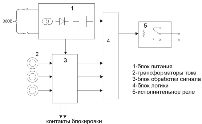
Рис. 2 Структурная схема
