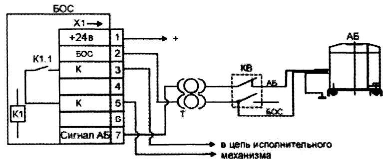
Схема электрических соединений прибора "Барьер-2000К"
