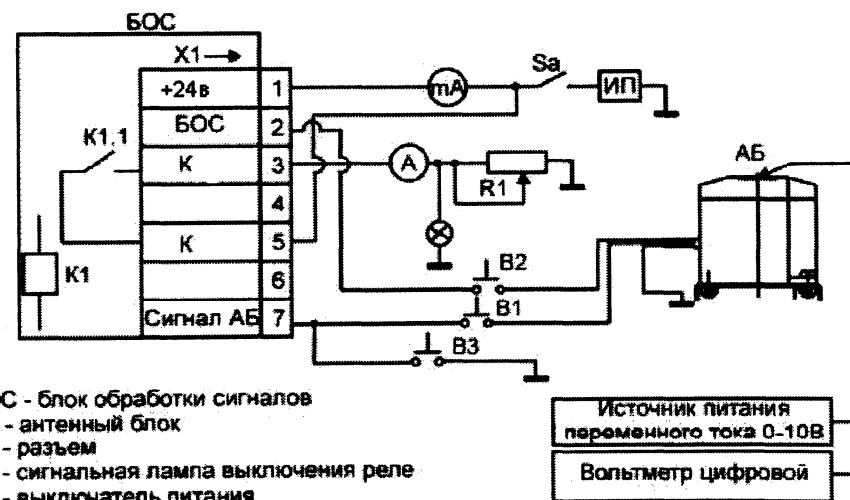
Электрическая схема стенда для проверки прибора "Барьер-2000К"
